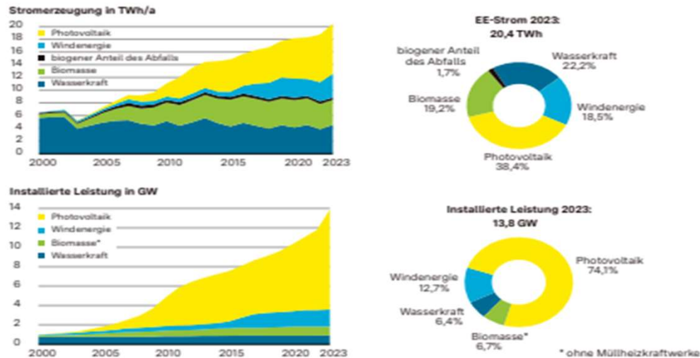
Entwicklung der Stromerzeugung aus erneuerbaren Energien und der installierten elektrischen Leistung in Baden-Württemberg
