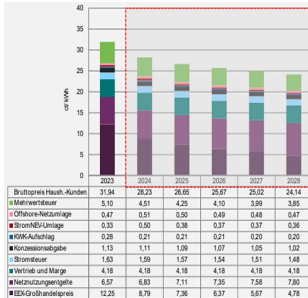
Abbildung 83 Reale Haushaltsstrompreise in Baden-Württemberg bis 2028
