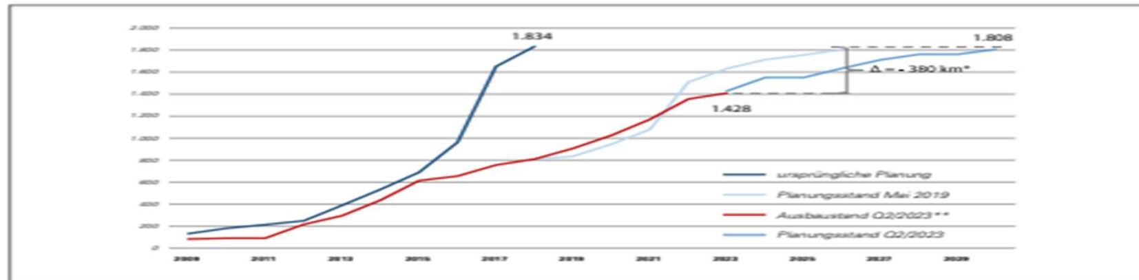
Abbildung 19: Ursprüngliche Planung, derzeitiger Ausbau- und Planungsstand der Netzausbauvorhaben gemäß EnLAG (Q2/2023).
