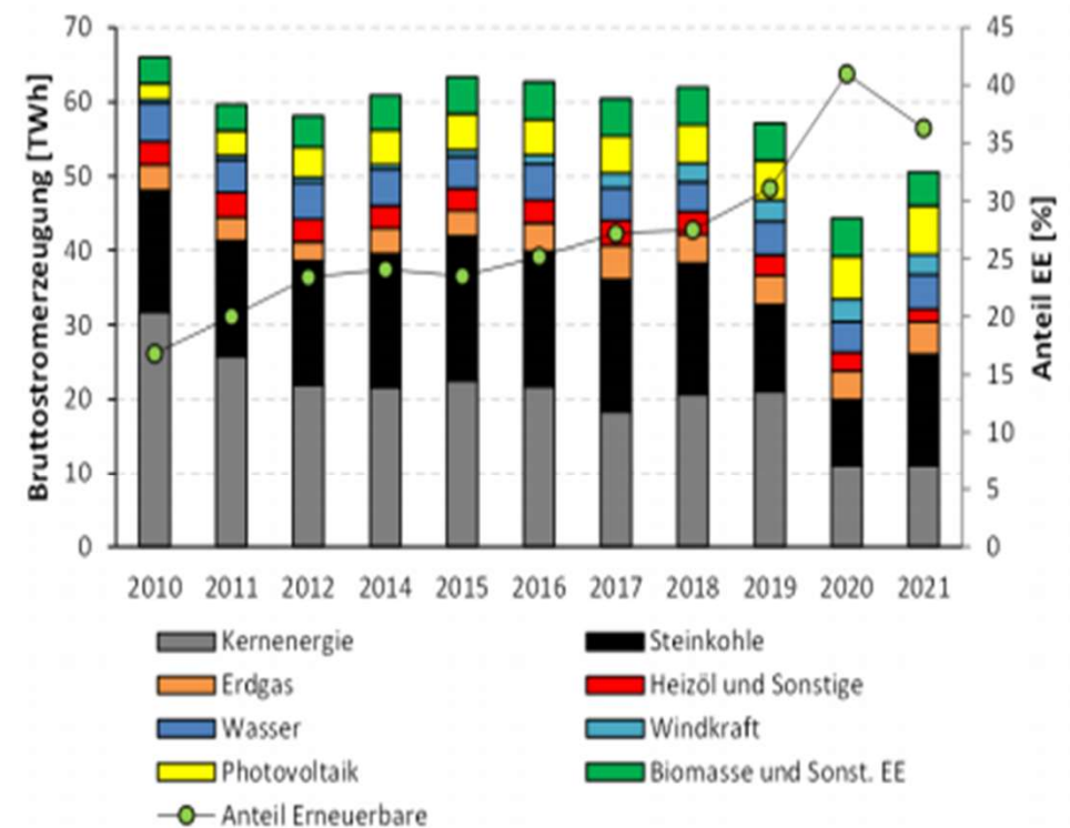
Abbildung 3: Entwicklung der Bruttostromerzeugung in Baden-Württemberg (Quelle: StaLa 2023)
