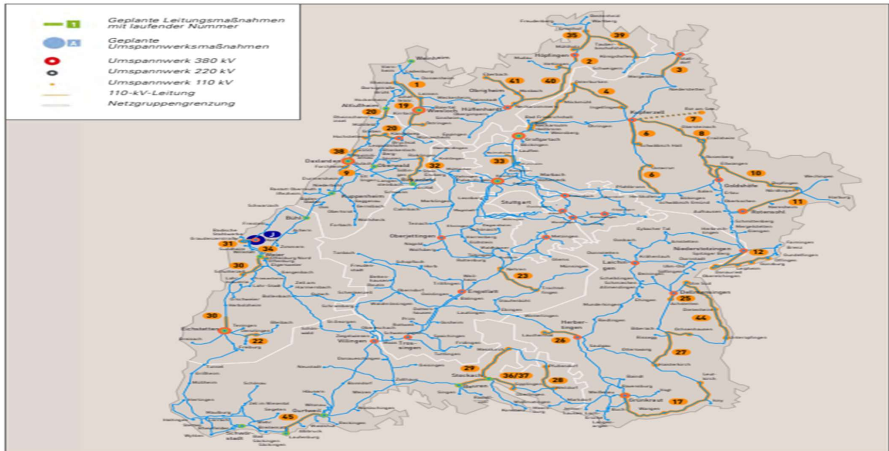
Abbildung 21: Geplante Netzverstärkungs- und Netzausbaumaßnahmen im Verteilnetz der Netze BW. Bearbeitete Darstellung basierend auf [164]
