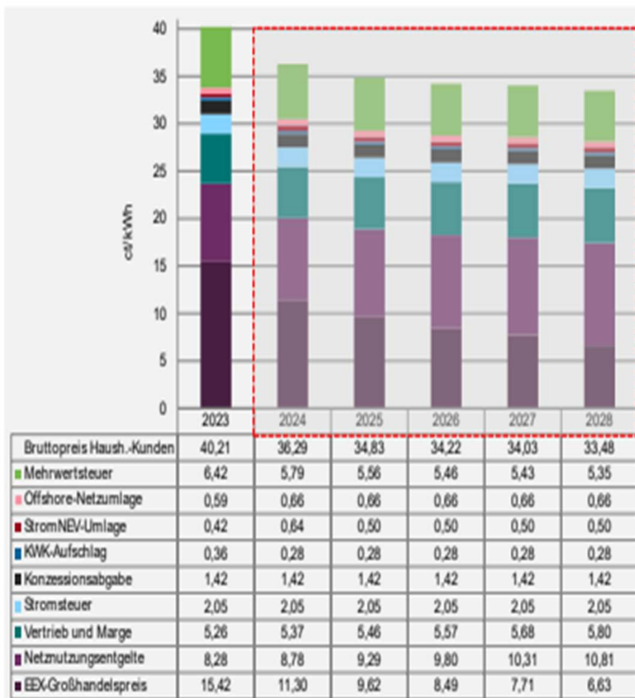
Abbildung 82 Nominale Haushaltsstrompreise in Baden-Württemberg bis 2028
