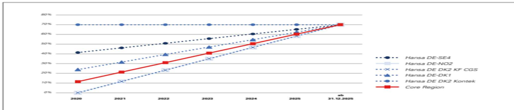
Abbildung 20: Lineare Pfade der festgelegten Mindestkapazitäten für den gebotszonenübergreifenden Stromhandel bis zum Jahr 2025. Eigene Darstellung basierend auf [160]
