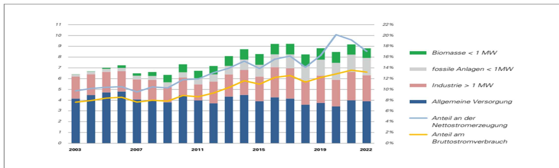
Abbildung 38: Entwicklung der KWK-Nettostromerzeugung nach Erzeugungsbereichen und des KWK-Anteils in Baden-Württemberg. Eigene Darstellung auf Basis von Daten aus [227–229] sowie eigenen Berechnungen. 2022 vorläufig.
