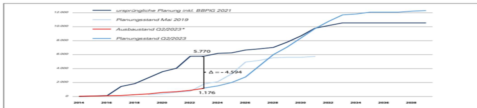
Abbildung 17: Ursprüngliche Planung, derzeitiger Ausbau- und Planungsstand der Netzausbauvorhaben gemäß BBPIG (Q2/2023)
