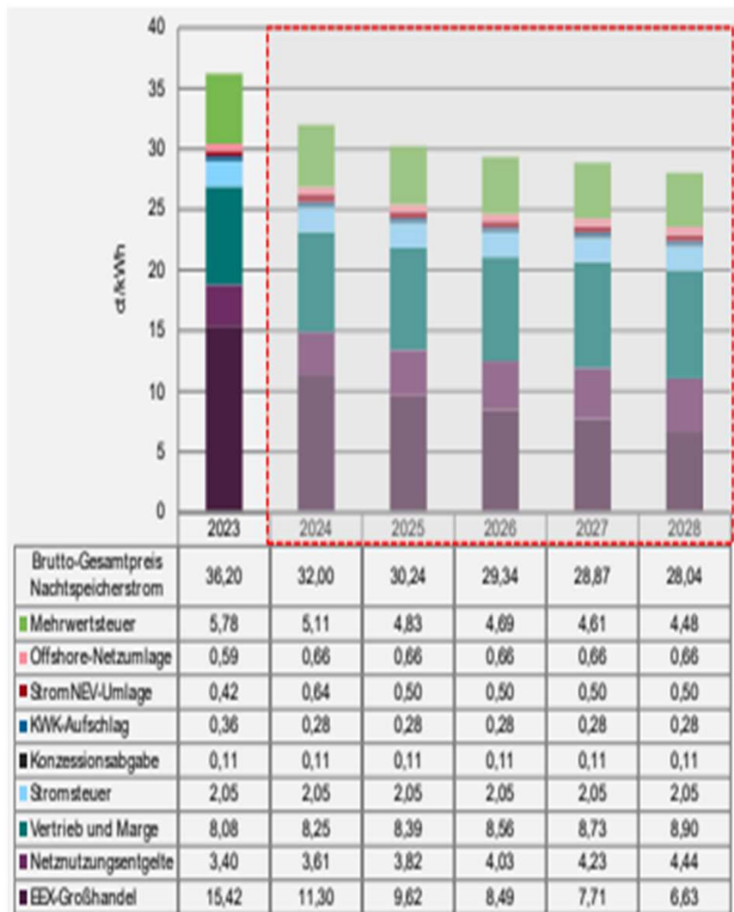
Abbildung 86 Nominale Nachtspeicher-Strompreise in Baden-Württemberg bis 2028
