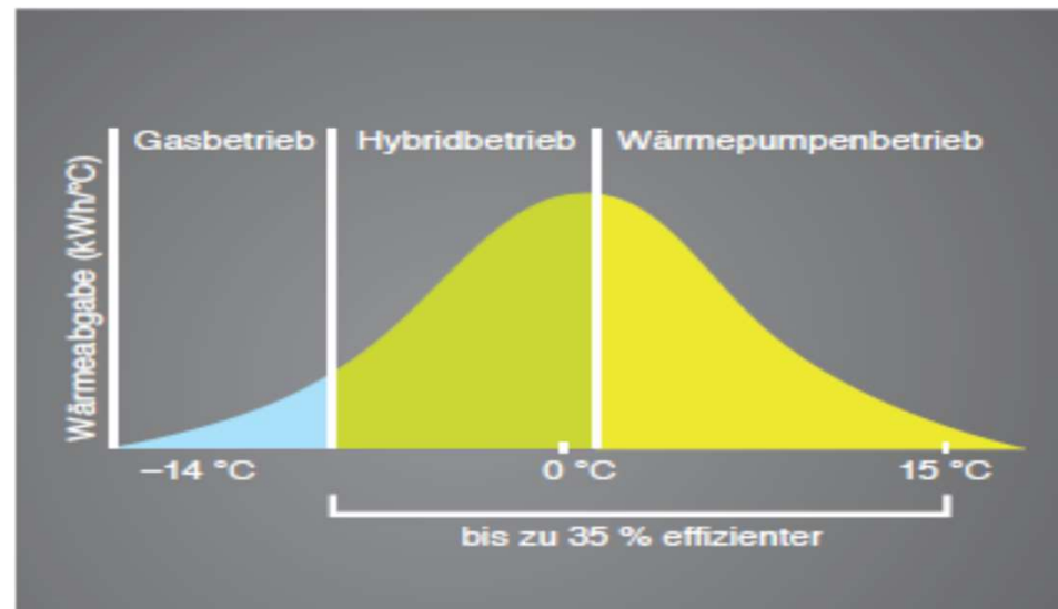
Abb. 35: Das hybride Wärmepumpensystem wählt automatisch die effizienteste Betriebsweise
