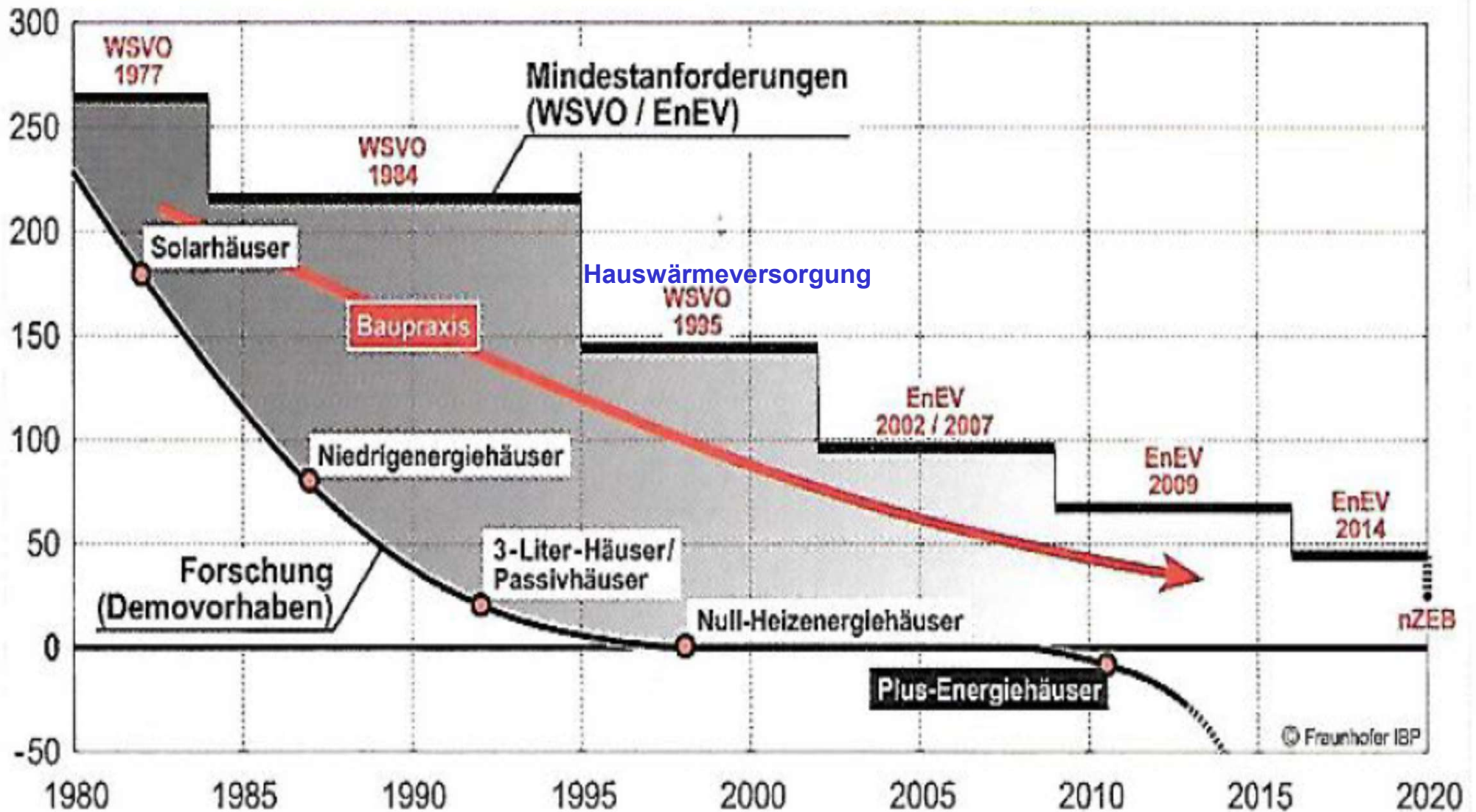
Primärenergiebedarf Doppelhaushälfte – Heizung [kWh/m 2 a]
