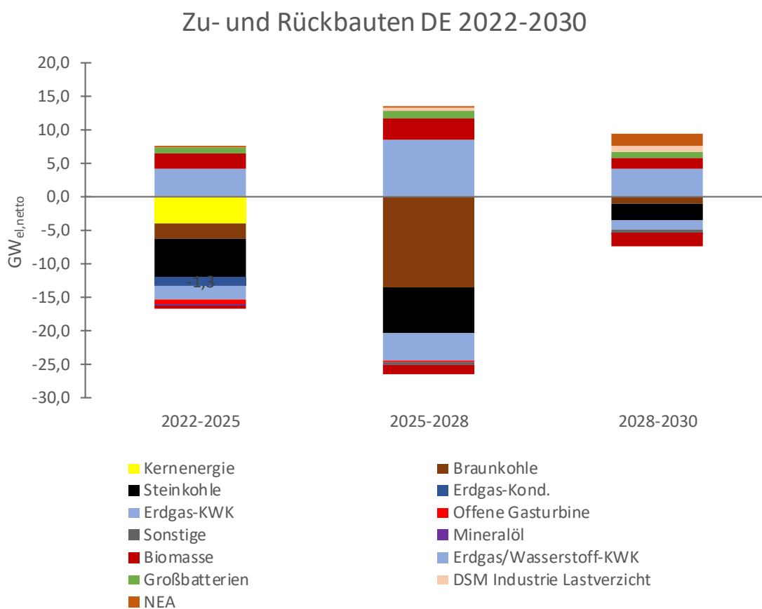
Abbildung 47 Rück- bzw. Zubau von nicht erneuerbaren Kapazitäten im Marktgebiet Deutschland (DE) (Quelle: r2b energy consulting)
