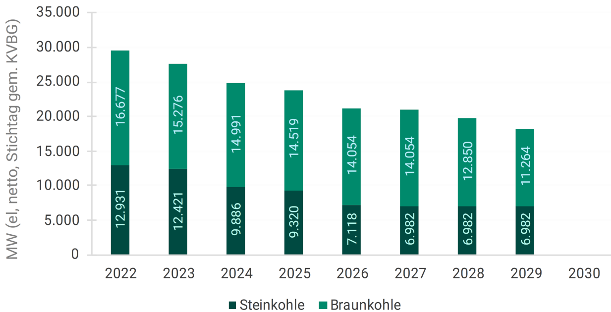
Abbildung 45 Entwicklung der maximalen Kohleleistung in Deutschland (Quelle: r2b)
