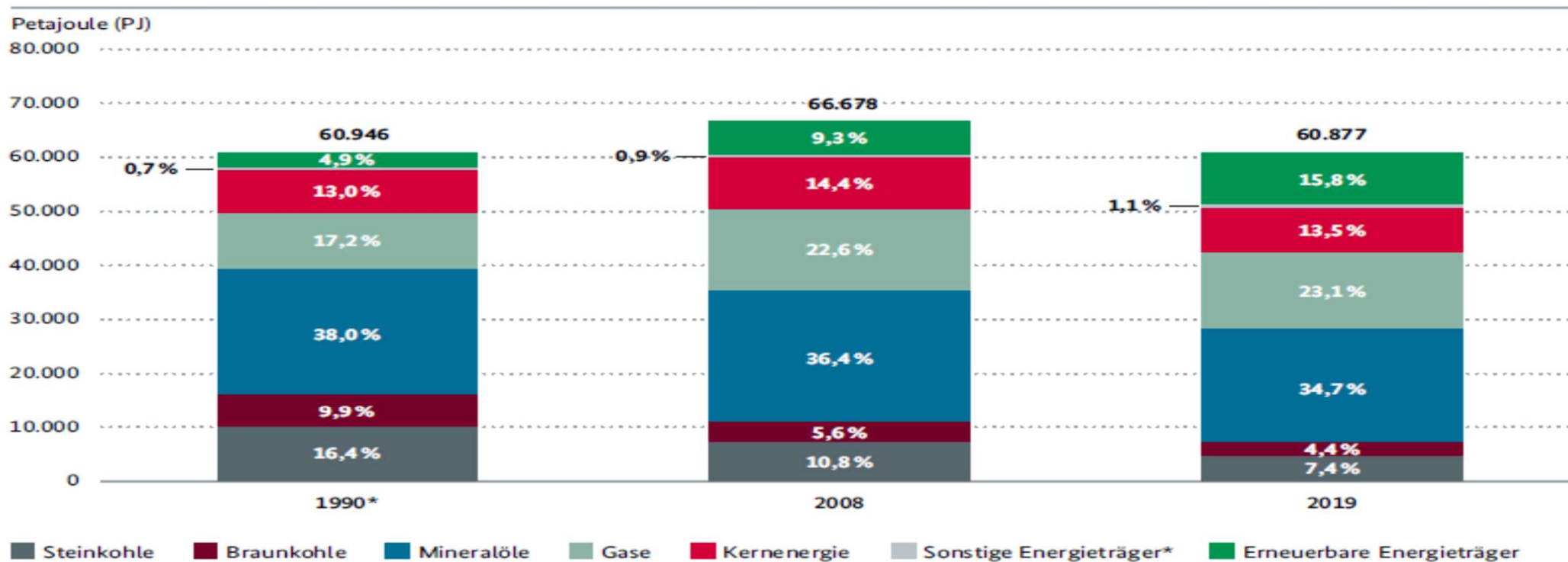
Abbildung 46: Primärenergiemix in der Europäischen Union (EU-27) 1990, 2008 und 2019 gemäß Bruttoinlandsverbrauch
