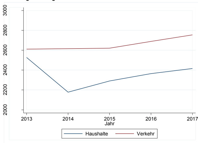
Abbildung 2: Entwicklung des Energieverbrauchs
