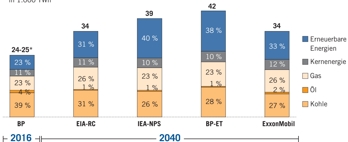
Abbildung 2.19: Synopse von Ergebnissen der EIA, IEA, BP und ExxonMobil zur weltweiten Stromerzeugung bis 2040
