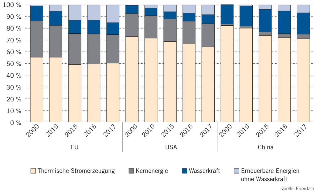
Abbildung 2.11: Entwicklung des Stromerzeugungsmix in der EU, den USA und China
