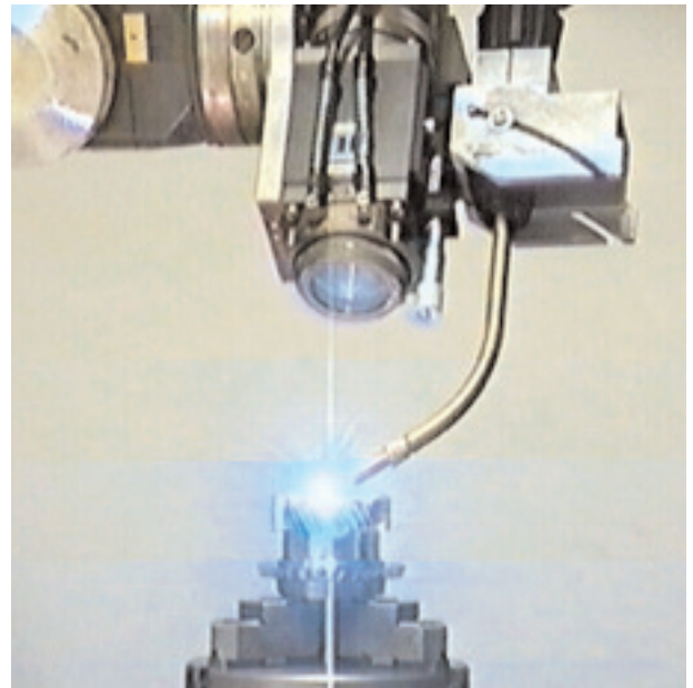
„Hightech“ Laserstrahlschweißprozess ohne Zugabe von Zusatzwerkstoff
